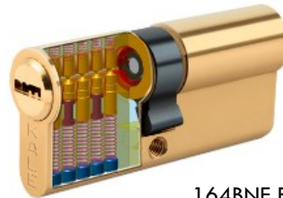
164BNE BALL BARREL
