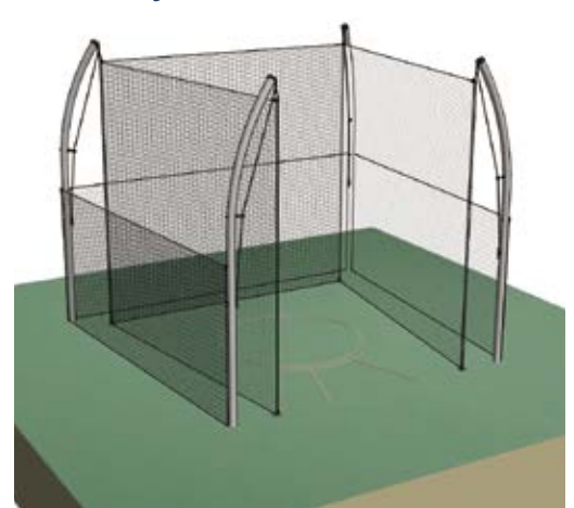
4 Pole Layout - SC-25BN
