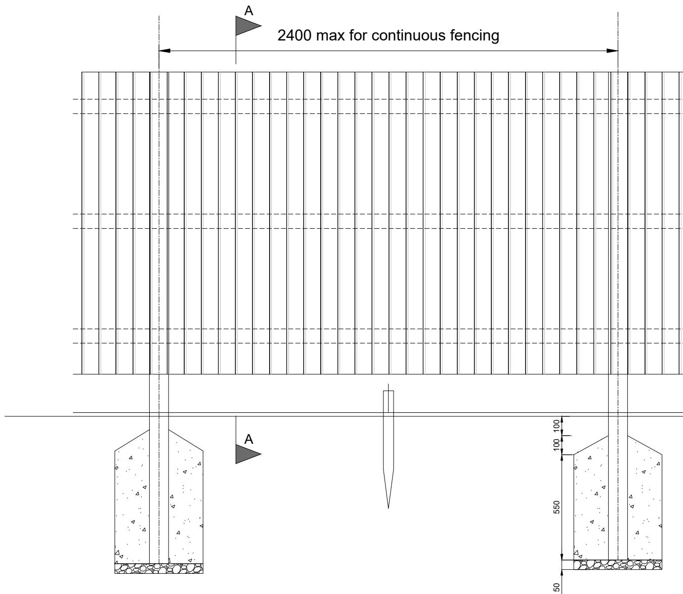
Elevation
