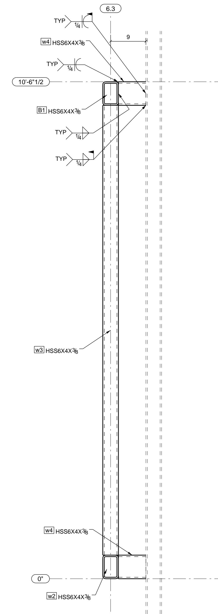
B - B SCALE: 1:12
