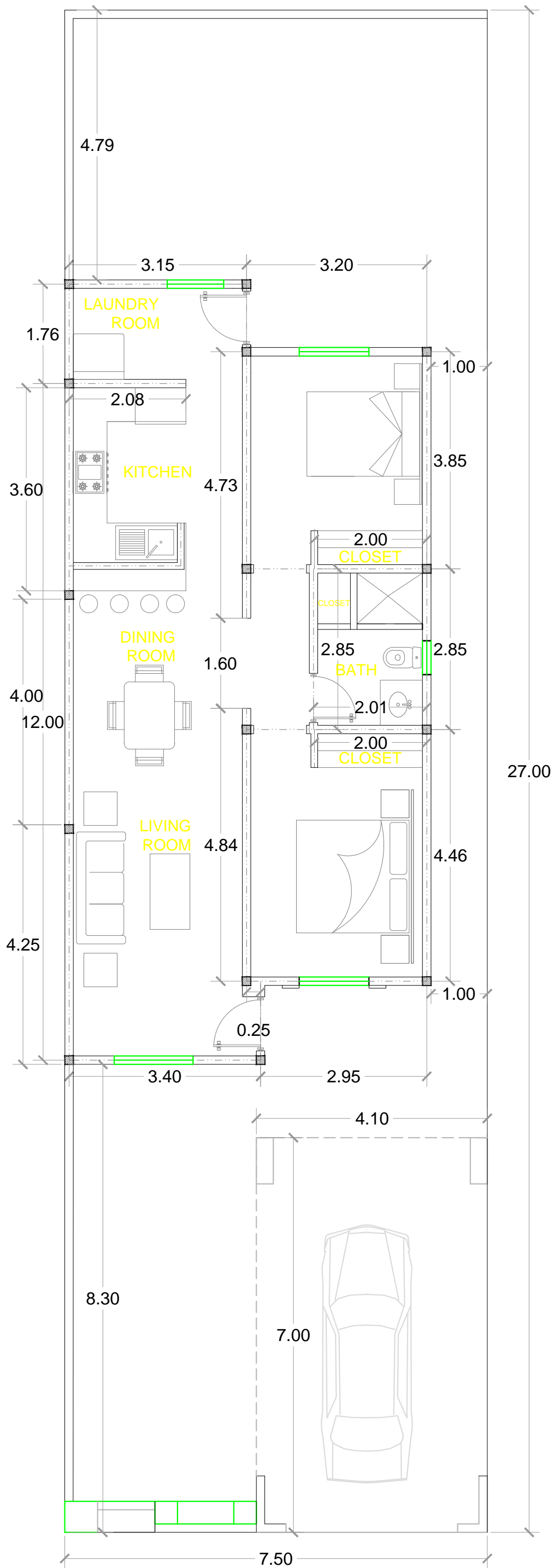
PLANTA ARQUITECTONICA 888 FT 2 LOTE 2180 FT 2
