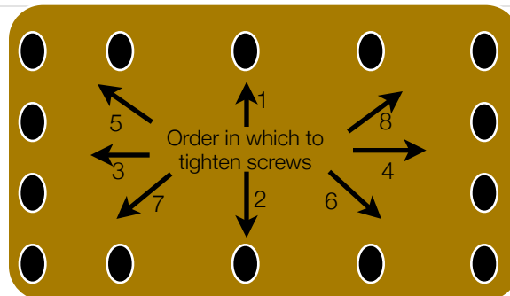
Enclosure Lid
