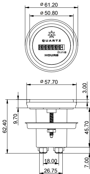
Cup Mount Bezel
