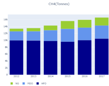
Figure 85 - a) CO 2 , b) CH 4 , c) N 2 O, d) NO x , e) CO, f) NMVOC, g) SO x ,h) PM 2.5 , i) PM, h) BC, delineated by HFO, MDO and NG
