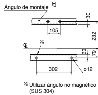
Troquelado en panel (vista frontal)
