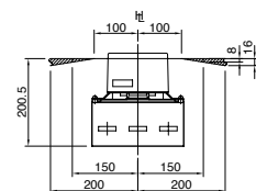
Posición de la bisagra del panel vista inferior (zona sombreada)
