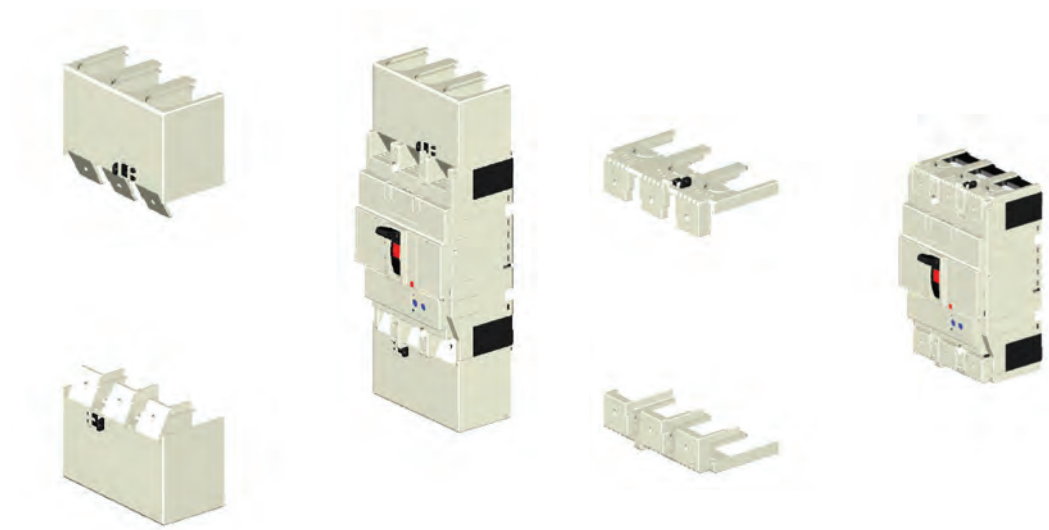
Tapas cubrebornes para conexión frontal
