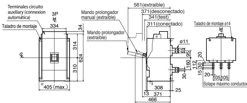
Extraíble
