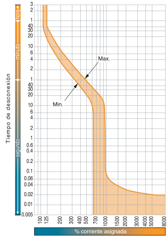
Curvas características tiempo/corriente S1000-ND
