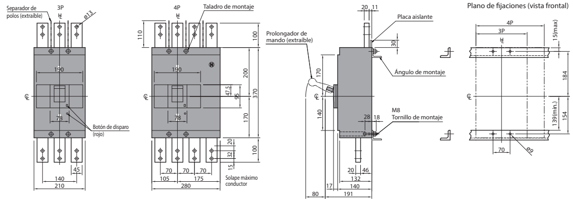
Conexión frontal
