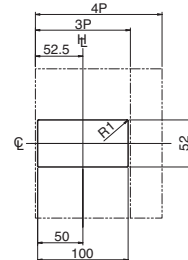
Troquelado en panel (vista frontal)
