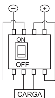
4 polos conectados en serie
