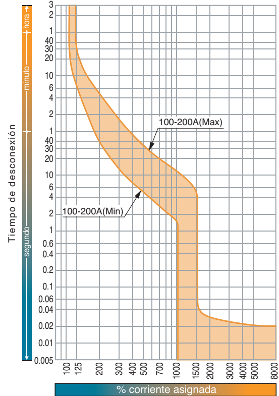
Curvas características tiempo/corriente S250-SD, S250 GD (100-200A)
