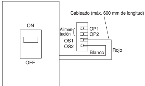
Fuente de alimentación del relé electrónico (OCR) instalado separado del interruptor
