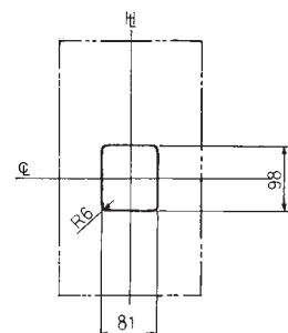
Troquelado en panel (vista frontal)
