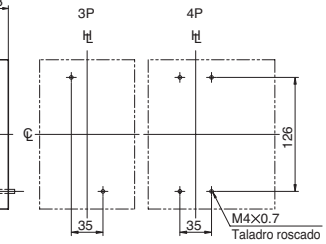
Plano de fijaciones (vista frontal)
