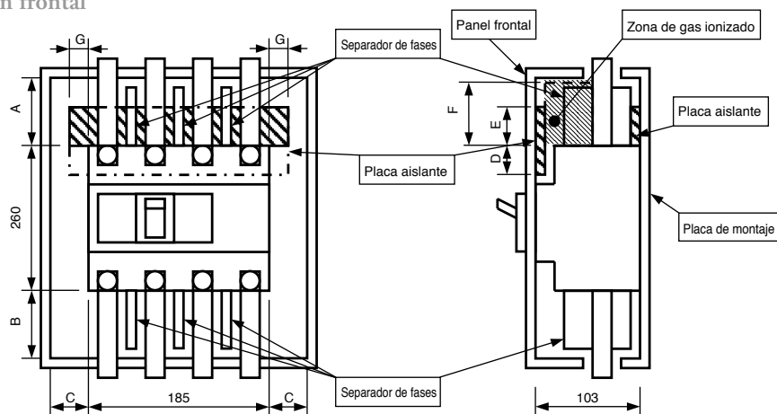
Conexión frontal
