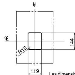
Troquelado en panel (vista frontal)
