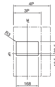
Troquelado en panel (vista frontal)
