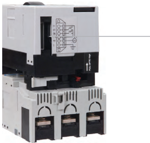
Interrupor y mando motor mostrando la toma para el conector de cables
