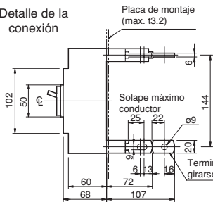
Conexión posterior
