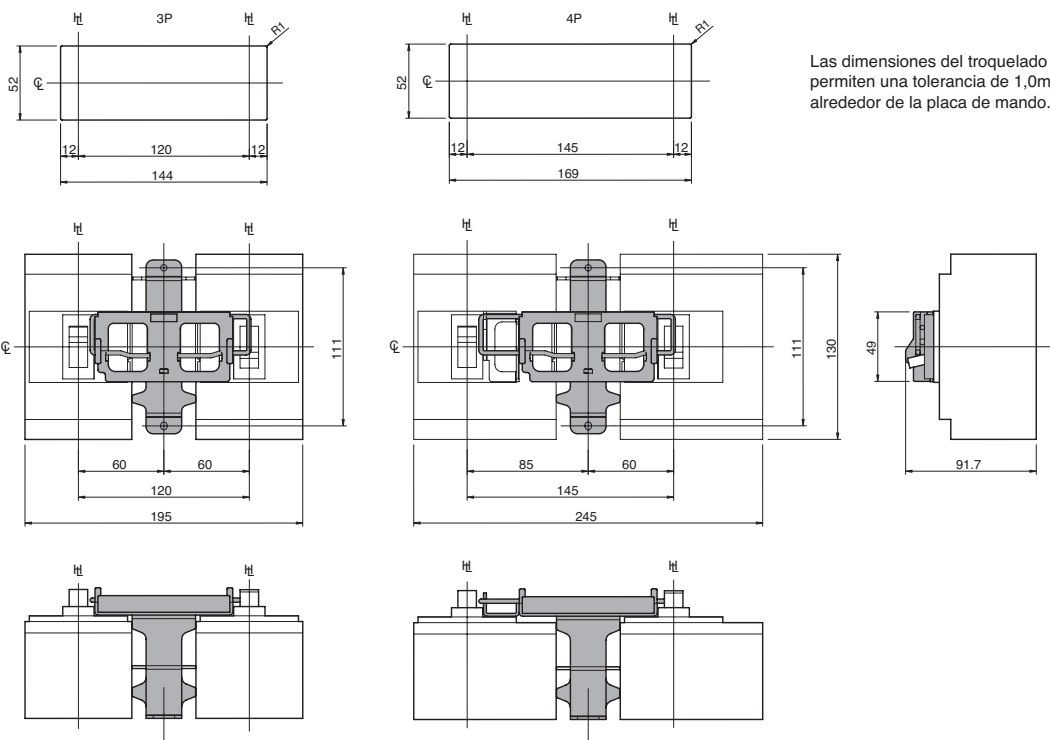
Plano de fijaciones (vista frontal)
