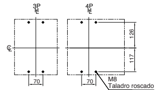
Plano de fijaciones (vista frontal)
