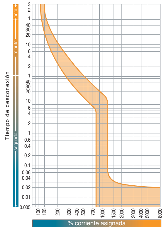
Curvas características tiempo/corriente S800-ND
