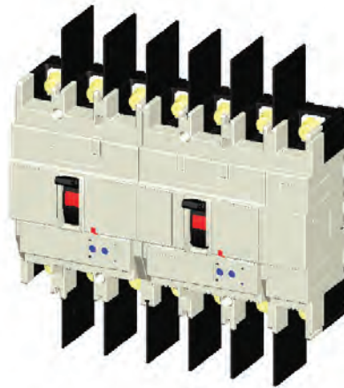
Separadores entre interruptores adyacentes
