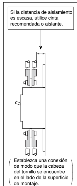
Conexión (dos cables eléctricos)
