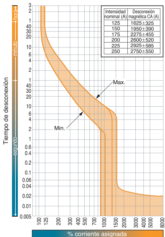
Curvas características tiempo/corriente E250-SCF, E250-SF, S250-SF
