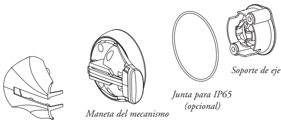
Tapa de la maneta
