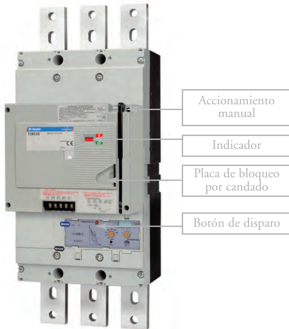
Mando motor tipo 1250 y 1600A
