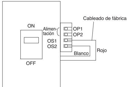
Fuente de alimentación del relé electrónico (OCR) instalado en el interruptor
