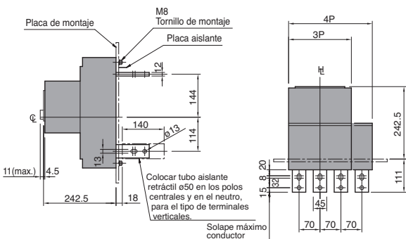
Conexión posterior con mando motor
