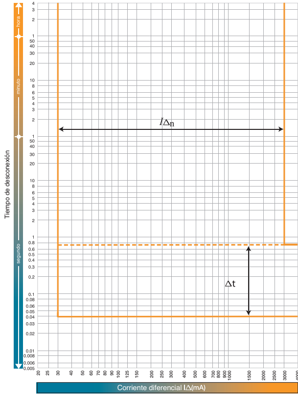
Curvas características tiempo/corriente ZE250-NJ, ZS250NJ, ZS 250-GJ, 160A
