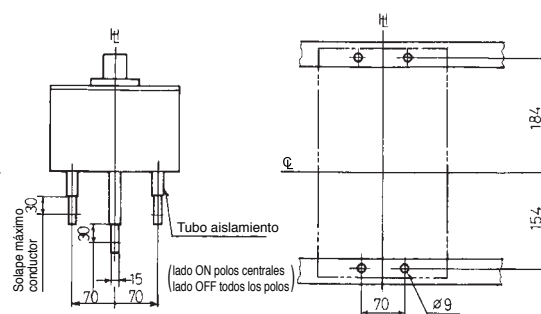
Plano de fijaciones (vista frontal)
