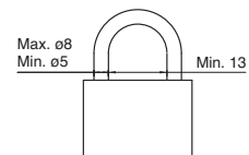
Dimensiones del candado (mm)
