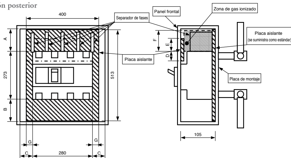
Conexión posterior
