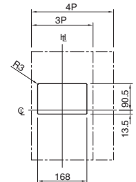
Troquelado en panel (vista frontal)
