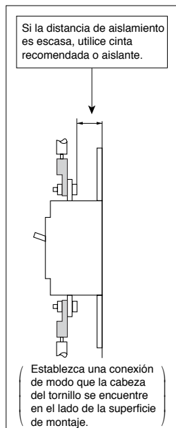
Conexión (un cable eléctrico)
