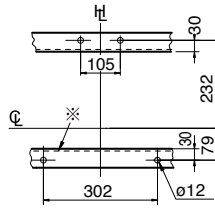
Plano de fijaciones (vista frontal)
