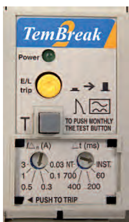
Pulsador de prueba, indicador de desconexión, LED de presencia de tensión y dial de ajuste
