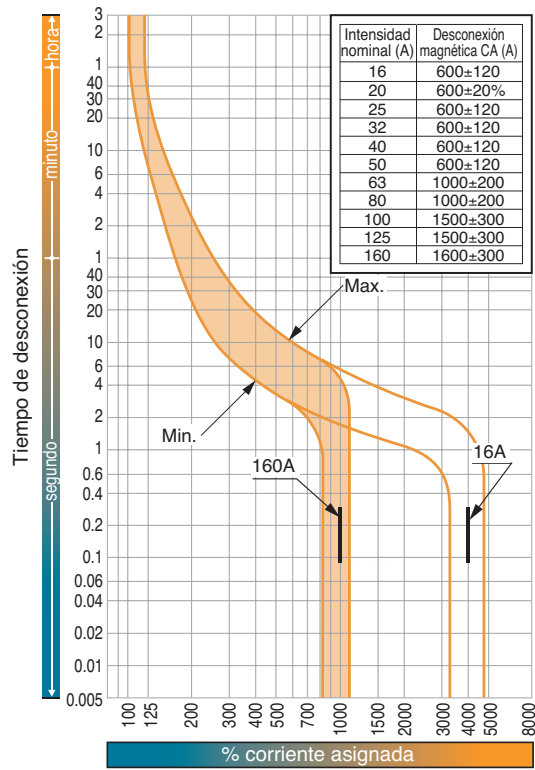
Curvas características tiempo/corriente E160-SF, S160-SCF, S160-SF
