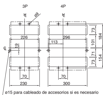
Plano de fijaciones (vista frontal)
