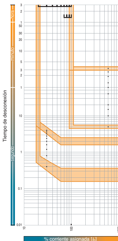
Protección de rotación de fase y alarma previa
