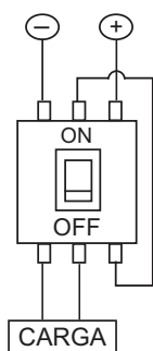
3 polos conectados en serie
