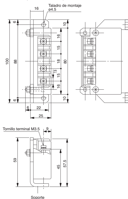
Fuente de alimentación del relé electrónico (OCR) instalado separado del interruptor
