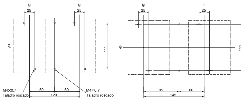
Plano de fijaciones (vista frontal)
