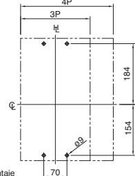
Plano de fijaciones (vista frontal)
