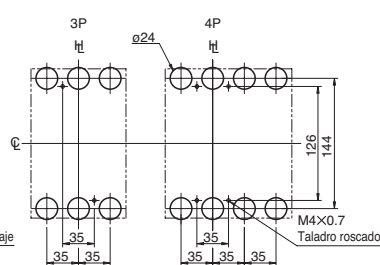
Plano de fijaciones (vista frontal)
