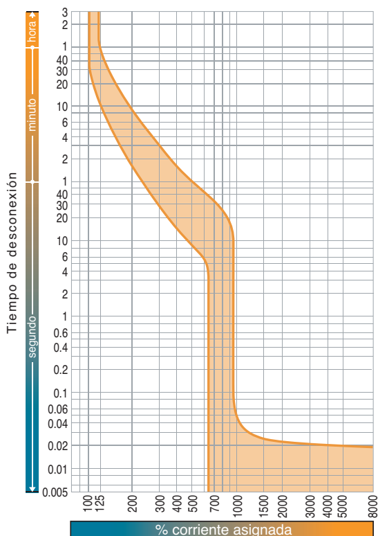
Curvas características tiempo/corriente PVS400-NDH PVS400-NDL 3P
