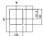
Troquelado en panel (vista frontal)
