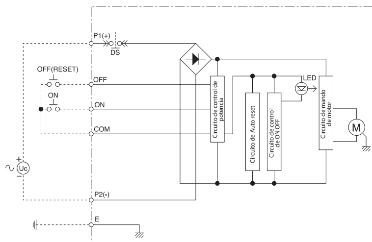
Circuitos de control para mando motor
