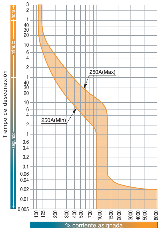
Curvas características tiempo/corriente S250-SD, S250-GD, (250A)
