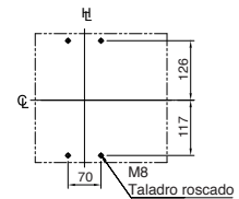
Plano de fijaciones (vista frontal)
