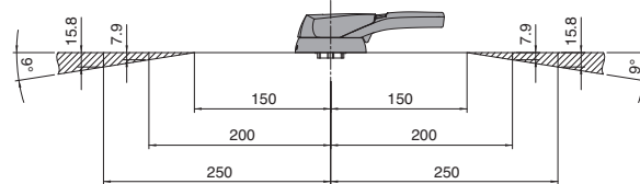
Dimensiones del candado (mm)
