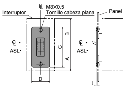
Plano de fijaciones del panel
