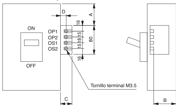
Fuente de alimentación del relé electrónico (OCR) instalado en el interruptor
