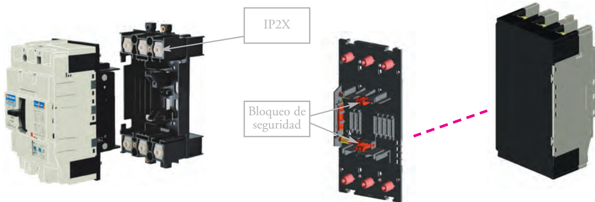
Interruptor enchufable y base
