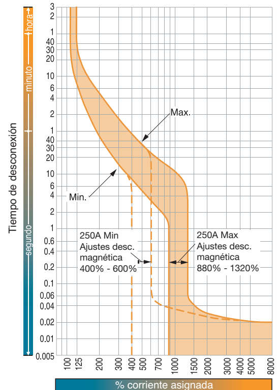
Curvas características tiempo/corriente E250-SCJ, E250-SJ, S250-SJ (250A)
