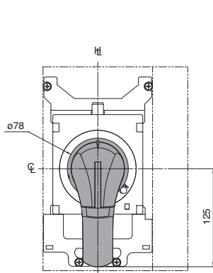
Troquelado en panel
