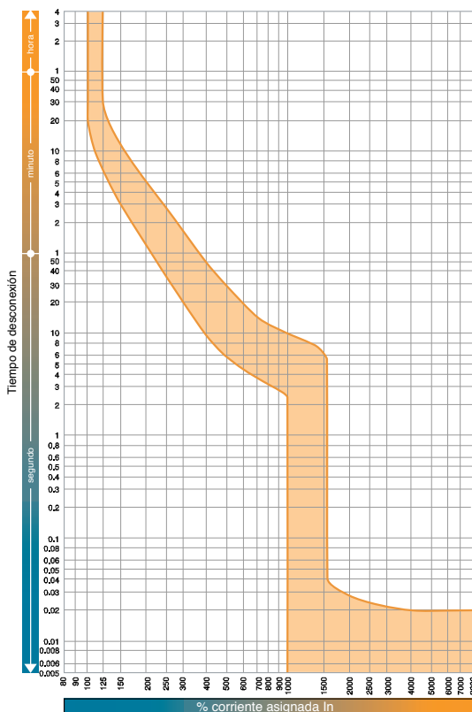
Curvas características tiempo/corriente ZE250-NJ, ZS250NJ, ZS 250-GJ, 160A
