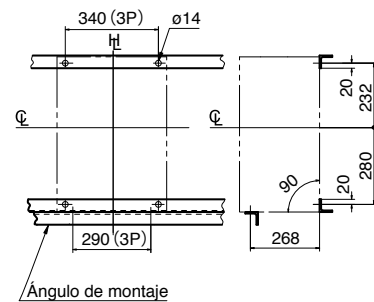
Plano de fijaciones (vista frontal)
