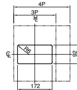
Troquelado en panel (vista frontal)
