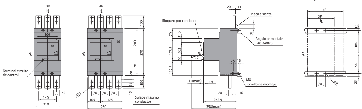
Conexión posterior con mando motor
