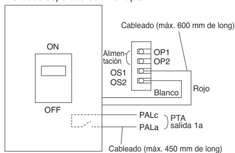
Fuente de alimentación del relé electrónico (OCR) instalado separado del interruptor
