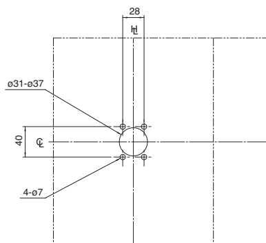
Troquelado en panel
