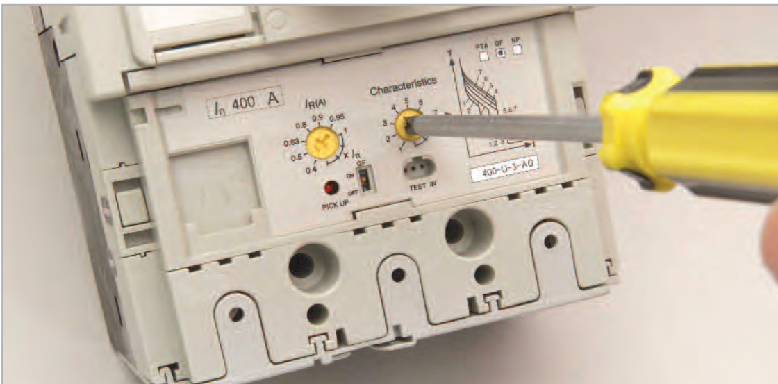
Seleccionando una característica predeterminada en un interruptor de 400A con protección electrónica
