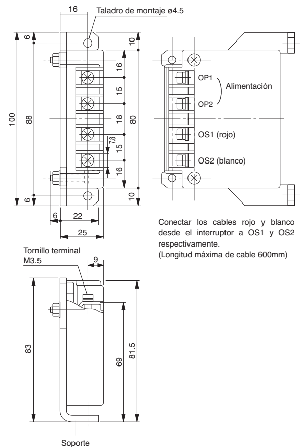
Fuente de alimentación del relé electrónico (OCR) instalado separado del interruptor
