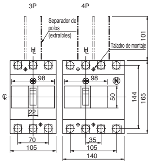
Conexión frontal
