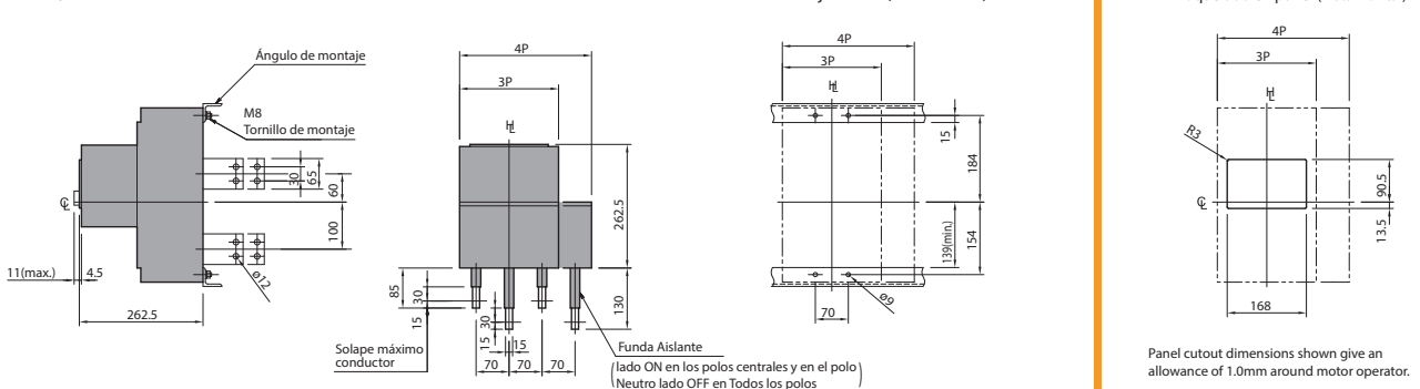
Conexión posterior con mando motor
