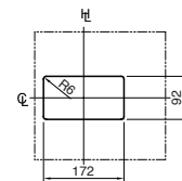
Troquelado en panel (vista frontal)
