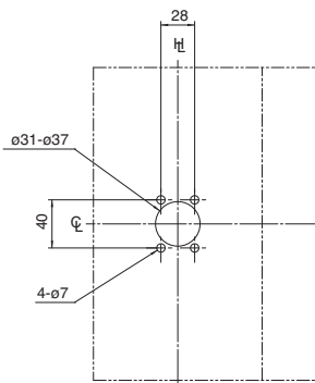
Troquelado en panel
