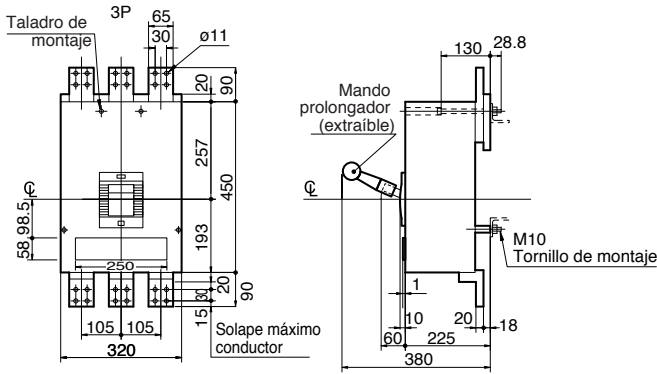
Conexión posterior
