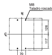
Plano de fijaciones (vista frontal)
