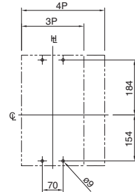
Plano de fijaciones (vista frontal)
