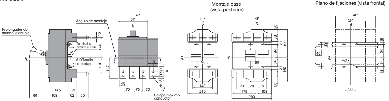
Enchufable
