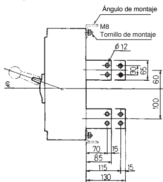
Conexión posterior
