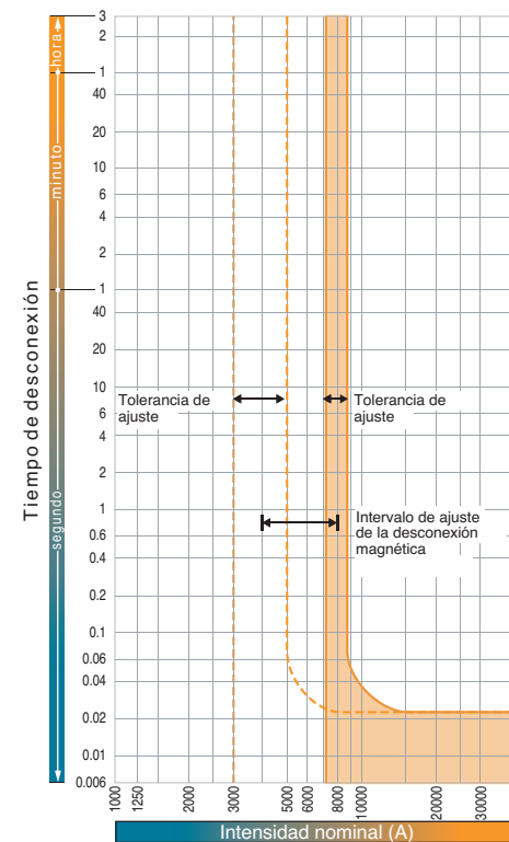
Curvas características tiempo/corriente XS1250ND, XS1600ND, XS2000ND, XS2500ND
