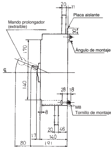
Plano de fijaciones (vista frontal)
