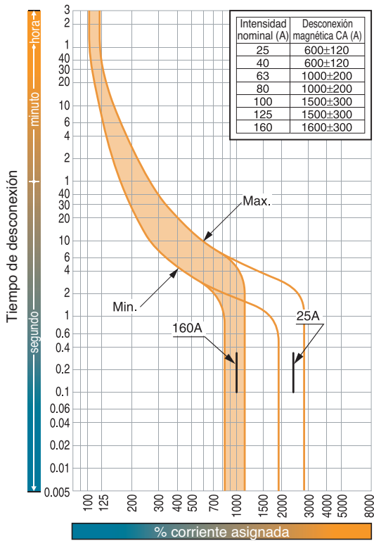
Curvas características tiempo/corriente E160-SJ, S160-SCJ, S160-SJ
