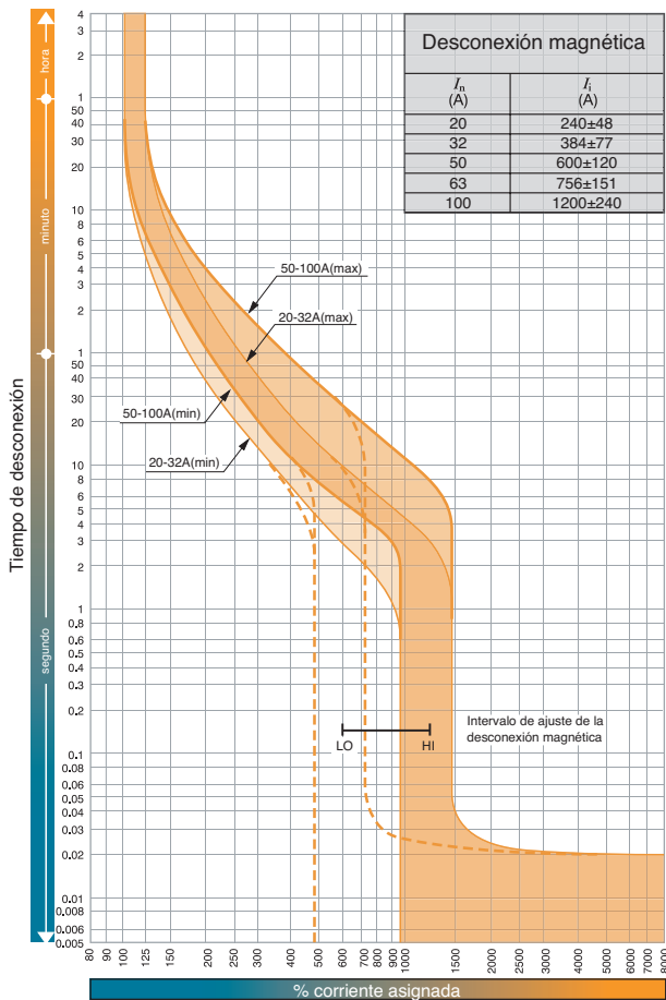
Curvas características tiempo/corriente S125-NJ, S125-GJ, VS125-NJ (20A a 100A)
