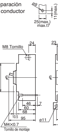
Con pletinas prolongadoras (opcional)
