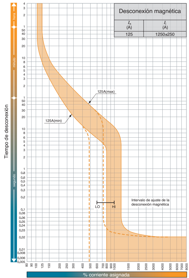
Curvas características tiempo/corriente S125-NJ, S125-GJ, VS125-NJ (125A)
