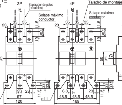
Con pletinas prolongadoras (opcional)
