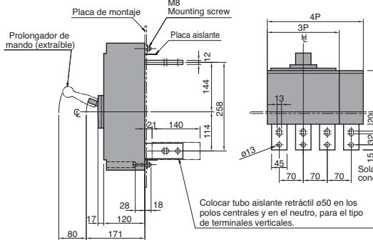
Conexión posterior
