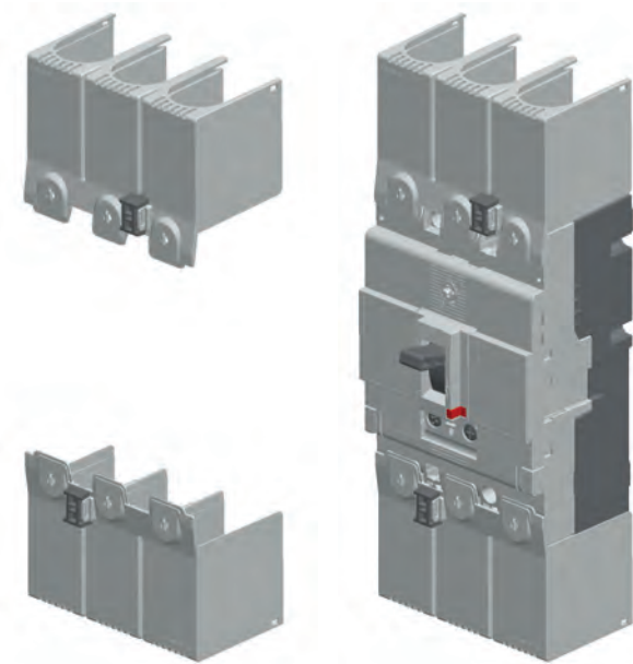
Tapas cubrebornes para conexión frontal (CF)
