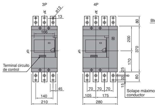
Conexión posterior con mando motor
