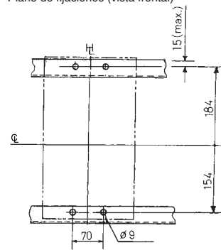
Plano de fijaciones (vista frontal)
