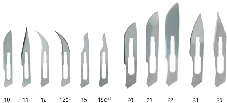
CS* SS** Size REF REF 4-110 4-310 10 4-111 4-311 11 4-112 4-312 12 4-112B Δ 4-312B Δ 12B Δ 4-115 4-315 15 4-115C ΔΔ 4-315C ΔΔ 15C ΔΔ
