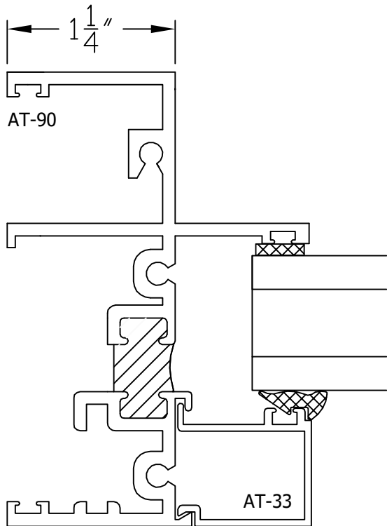
④ JAMB @ FIXED
