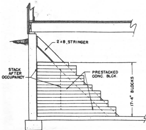
End Elevation
