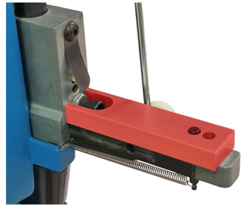
Installed on RL 550 Press Primer Slide.
