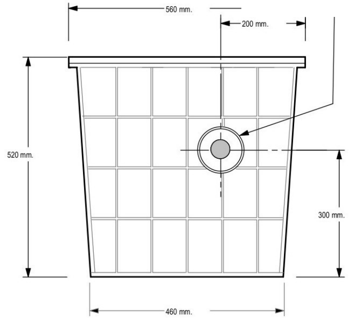
End Elevation
