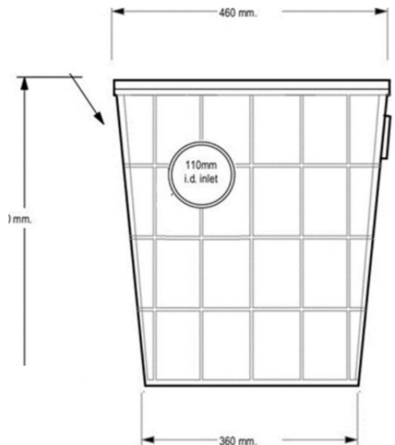
End Elevation
