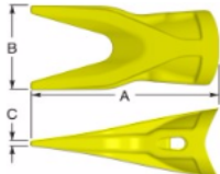
UT Twin Tiger
