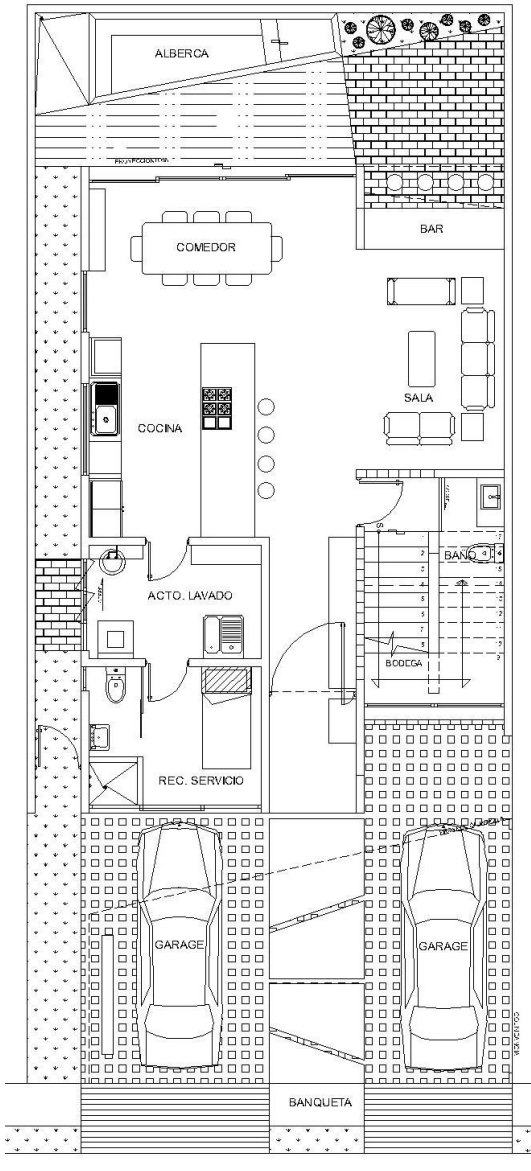
PLANTA BAJA
