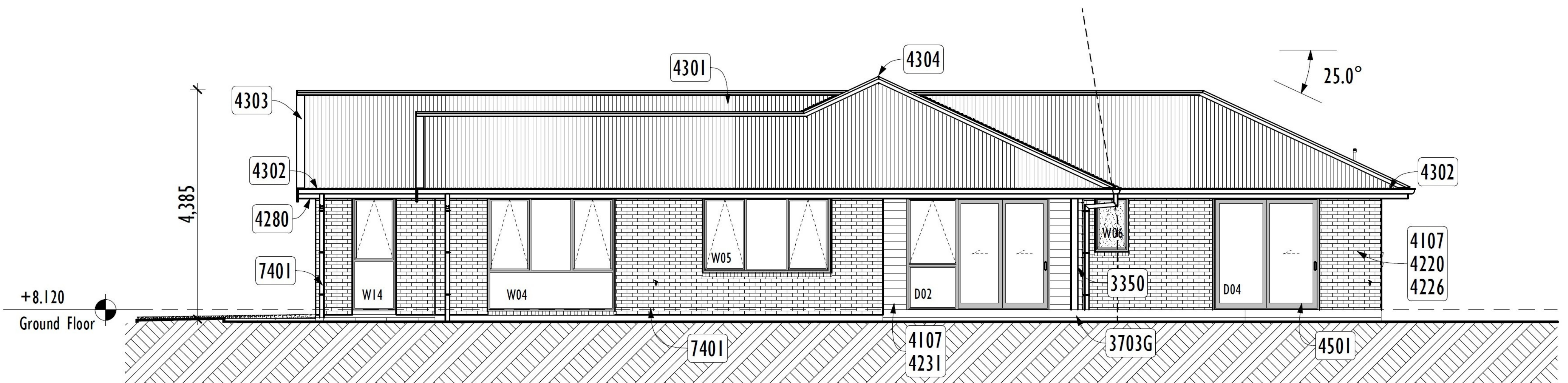
ELEVATION 3 1:100
