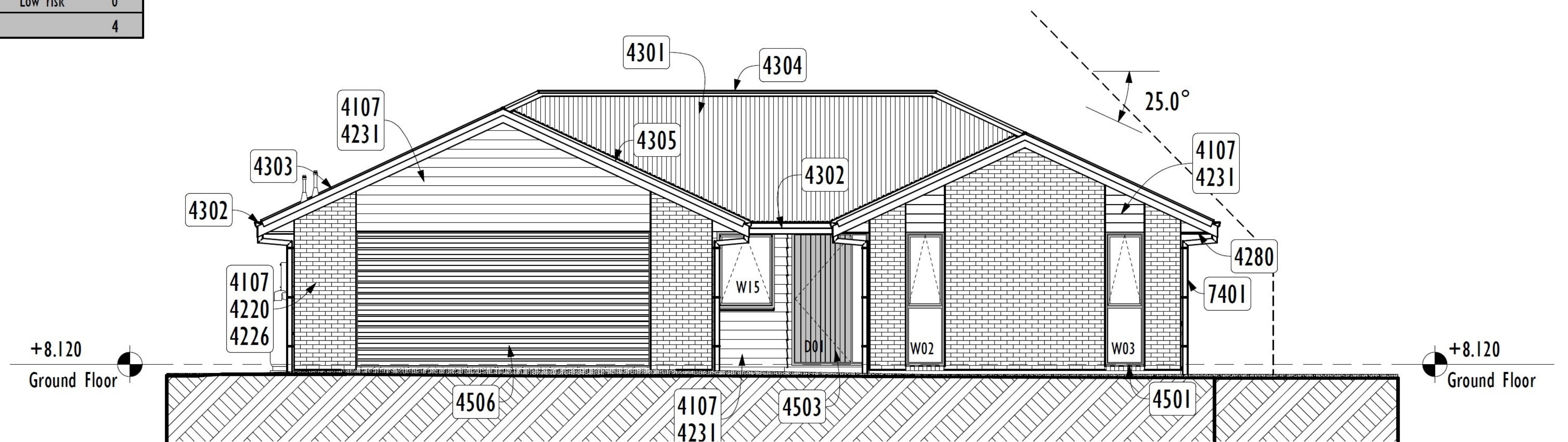
7 ELEVATION 2 1:100
