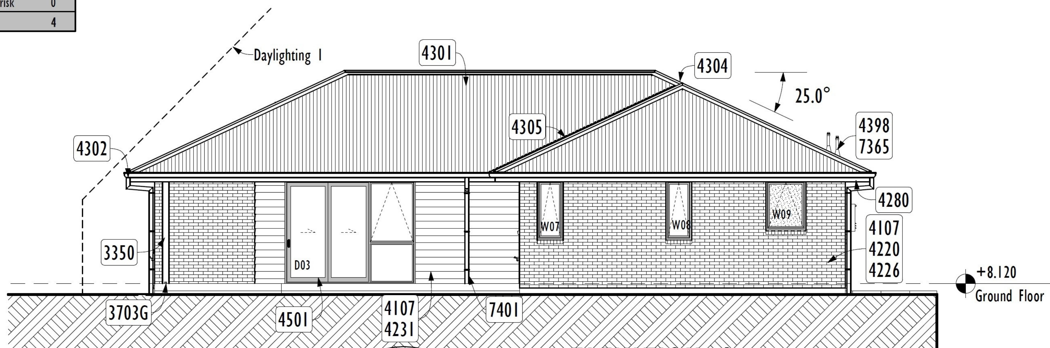
ELEVATION 4 1:100
