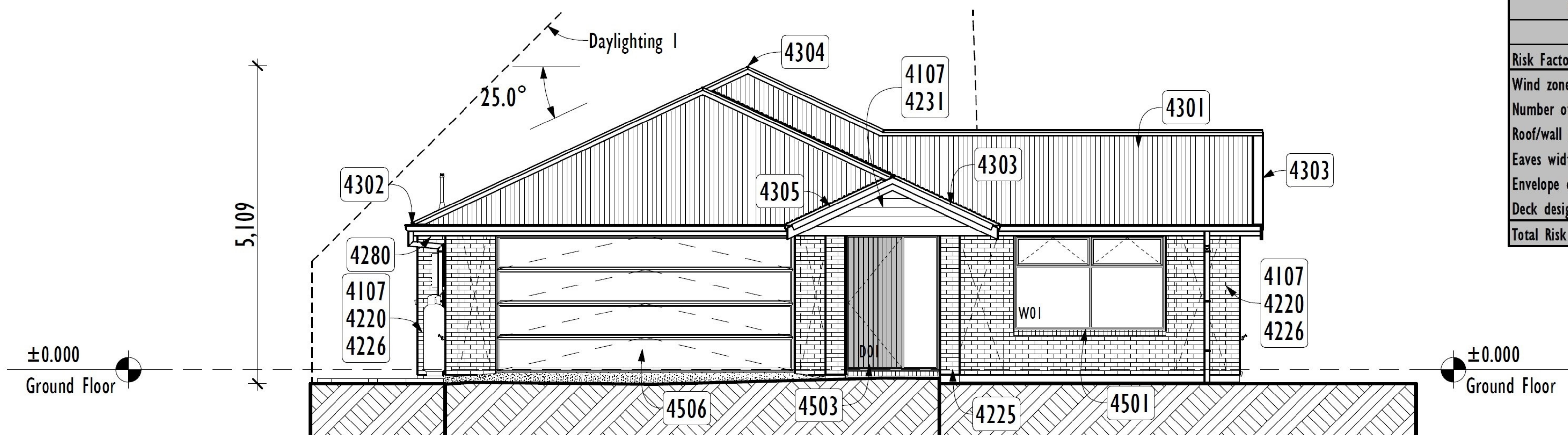
6 ELEVATION 2 1:100
