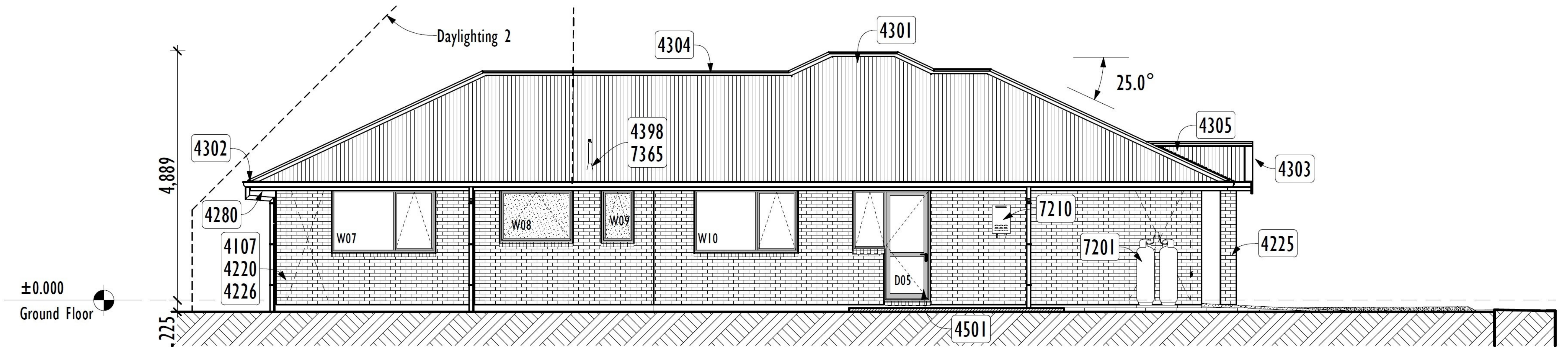
5 ELEVATION 1 1:100
