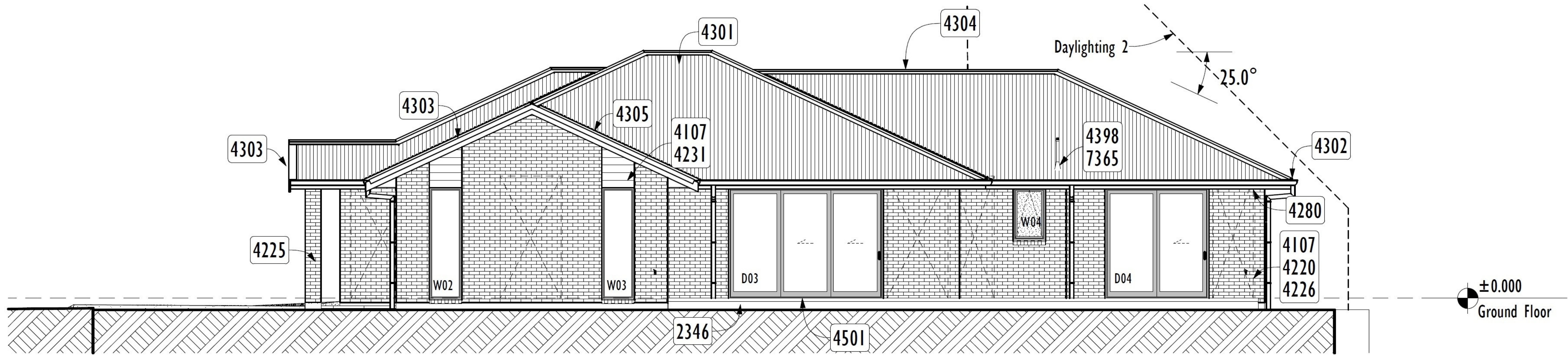
7 ELEVATION 3 1:100
