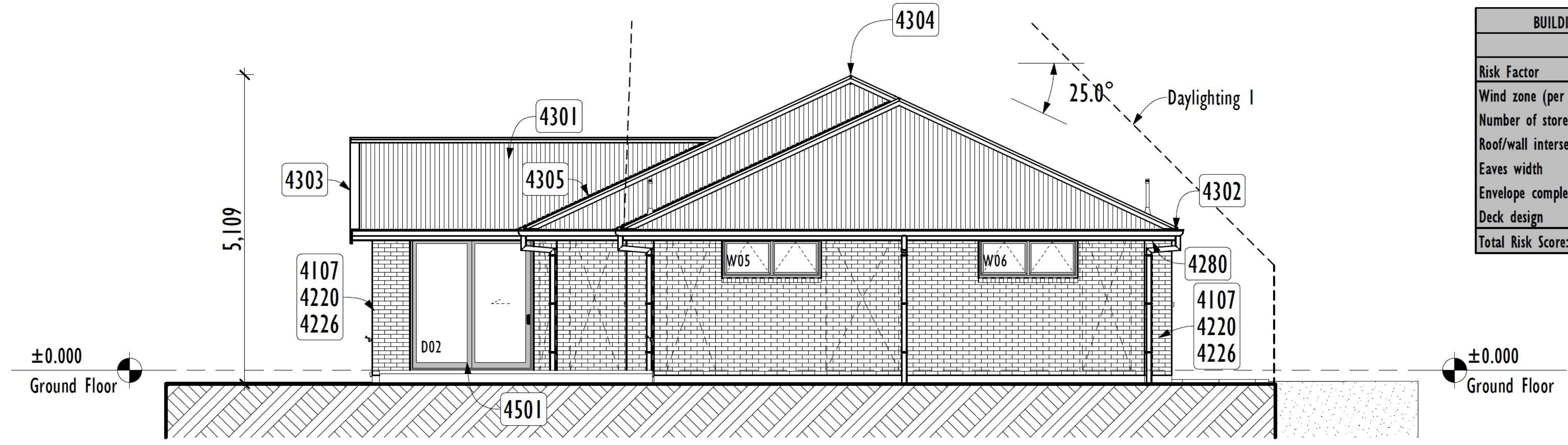
8 ELEVATION 4 1:100
