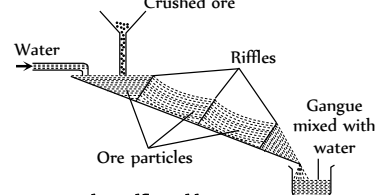
Fig. 16.1. The Wilfley table
