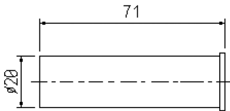
S8/035P Pin
