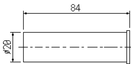
S8/030P Pin
