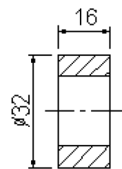
S8/031R Roller
