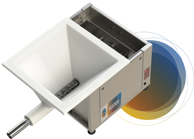
De Hethon Flexible Wall Hopper in een Feeder
