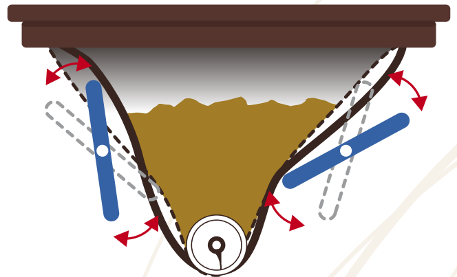
Het proces van de Hethon Flexible Wall Hopper
