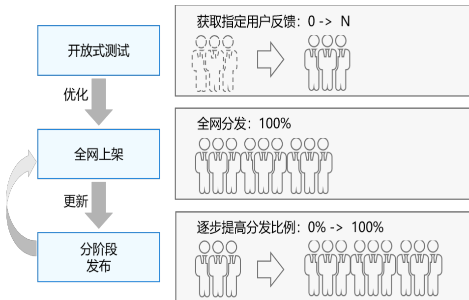
图 6-5: 分发阶段
