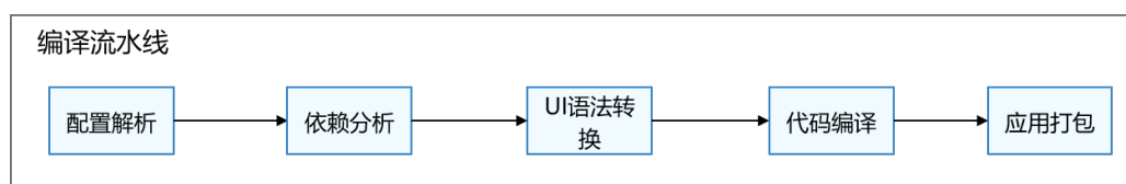
图 5-8：编译流水线
