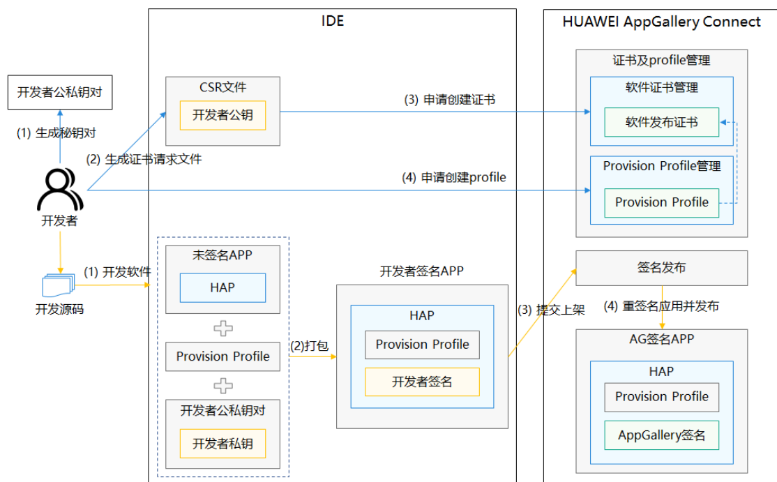
图 6-2: 签名方案
