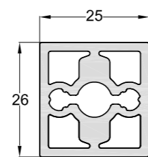
Traverso superiore e inferiore spalla Top and Bottom Horizontal Profile P10504
