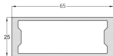
Profilo Anteriore Spalla Front Profile P10503
