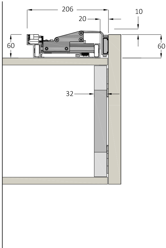
PENSILE CUPBOARD
