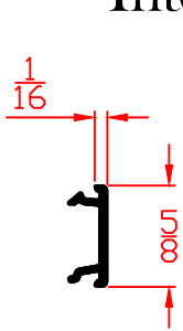
5839 1/2" Groove Filler
