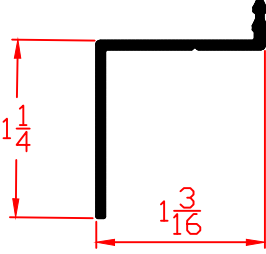
5945 4-9/16" Backset Windbreak
