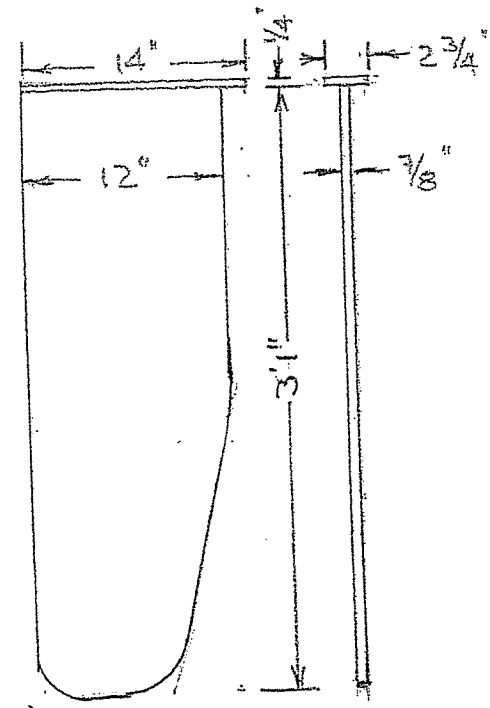
DAGGERBOARD
