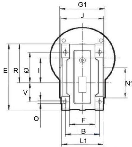
Input Flange
