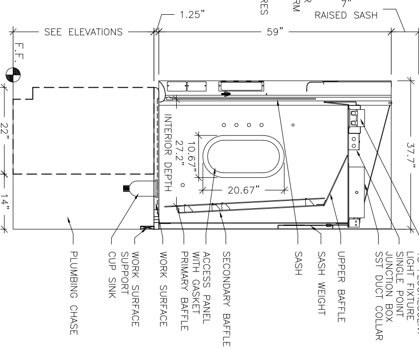
SIDE VIEW SCALE: 1/2" = 1'-0"
