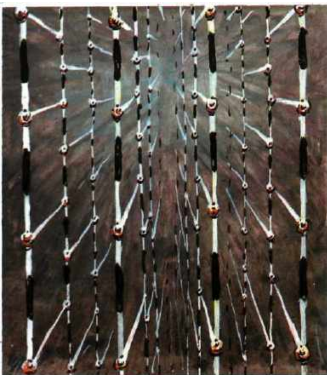
Фосфены — цветные подвижные узоры в глазах — можно вызвать воздействием на людей различных многополостных структур. Здесь — лишь некоторые из большой «коллекции» ЭПС-фосфенов.
