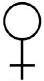
Venus
