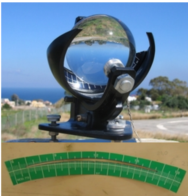
Figura 22. Heliógrafo para medida da insolação e fita de medição de horas de sol pleno durante um dia de céu limpo. Fonte: Adaptado de Wikipedia e IAG-USP.
