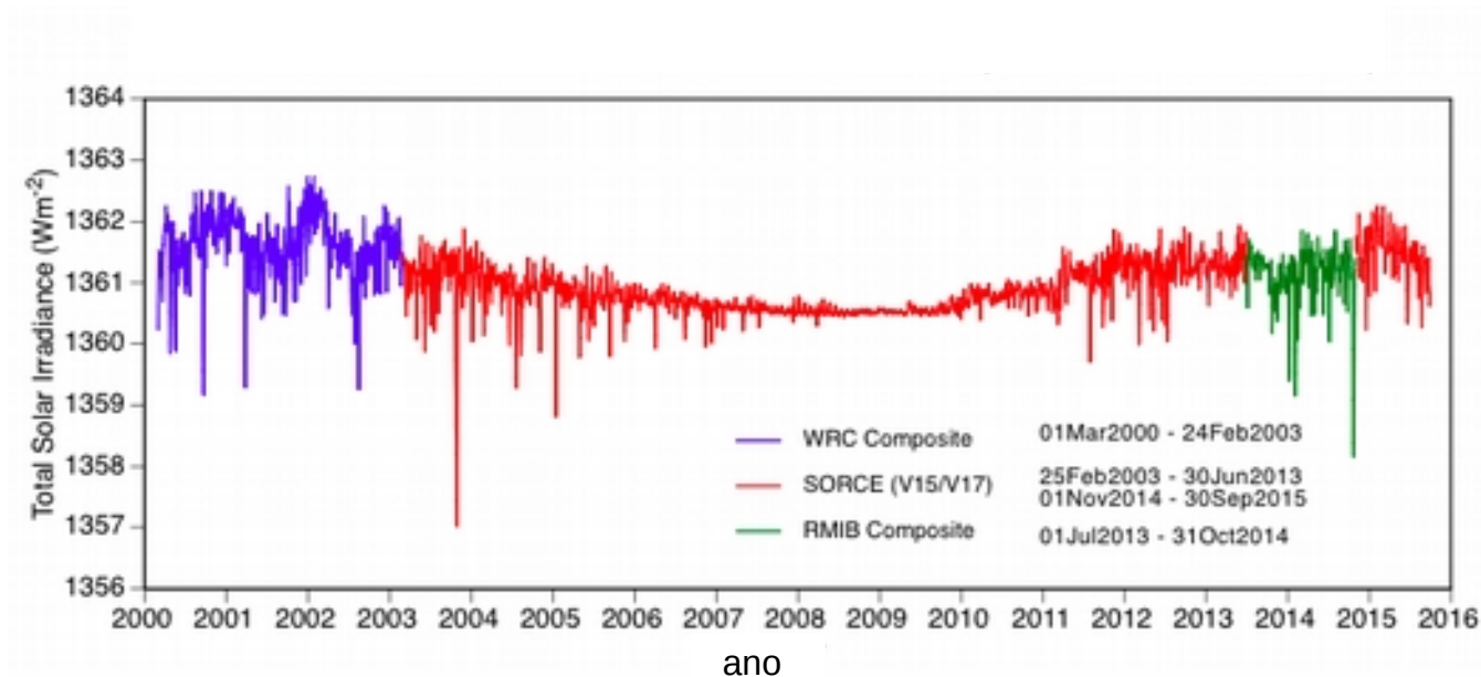
Figura 10. Valores da Irradiância Solar Total (TSI) entre 2000 e 2016. Compilado de NASA: https://ceres.larc.nasa.gov .
