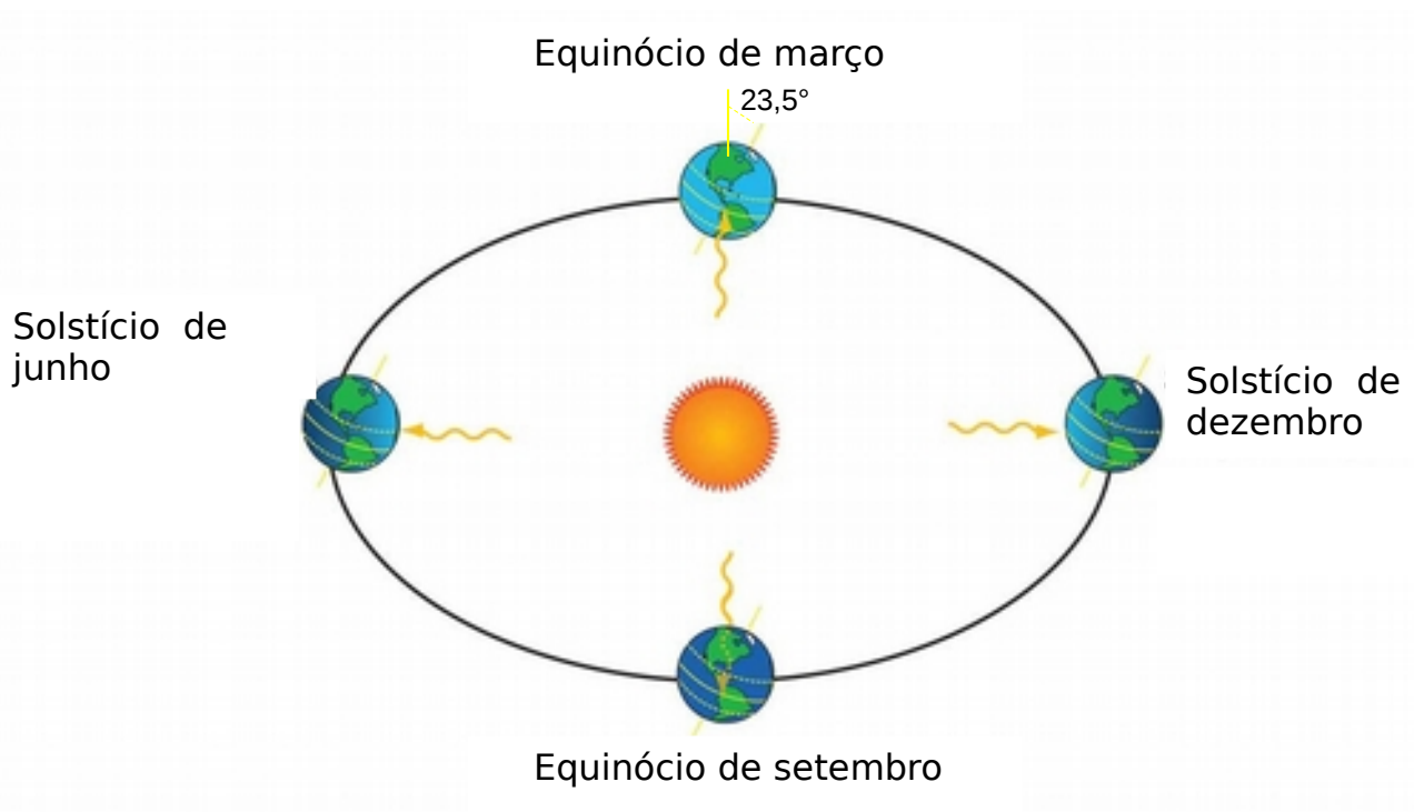
Figura 12. Estações do ano para o hemisfério Sul em função da inclinação do eixo de rotação e translação terrestre.
