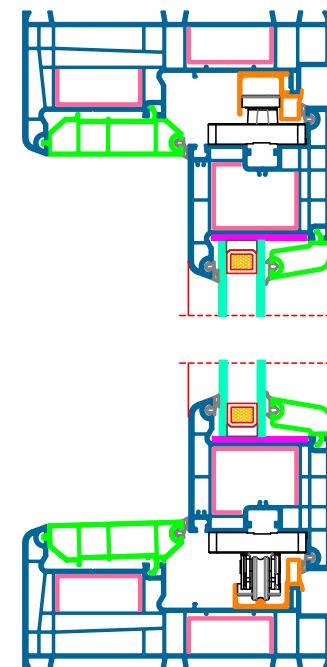
SECTION A-A
