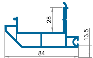
ESL 1825 Interlock Profile
