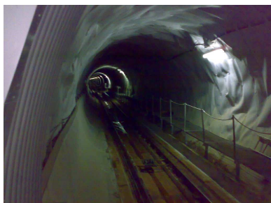
Tunnel du funiculaire de Bulnes – Espagne 2008 Tunnel de 2000 mètres avec un dénivelé de 18%.
