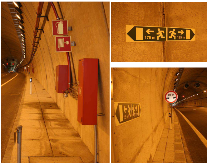
Tunnel routier A27 Viana de Castelo - Ponte de Lima - Portugal 2008
