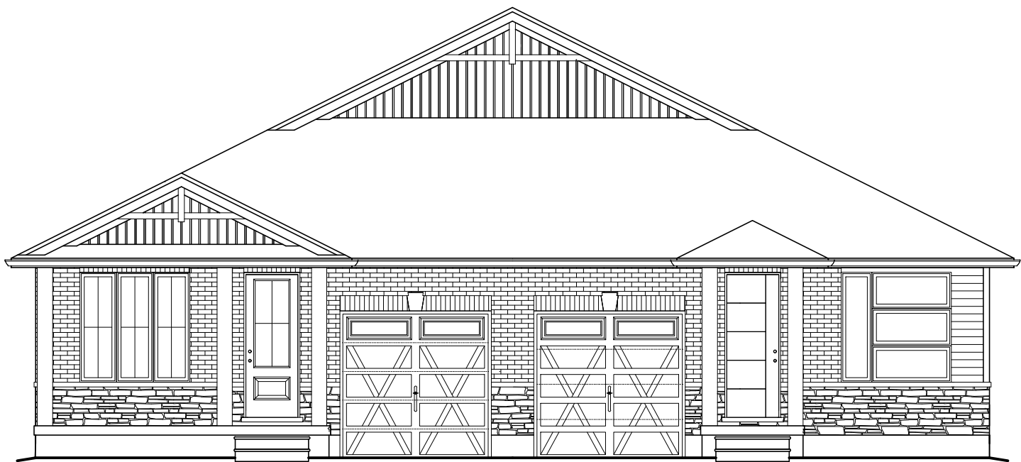
ELEV. A
