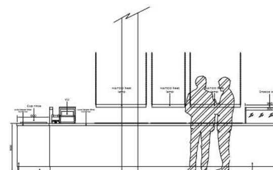
ELEVATION BB
