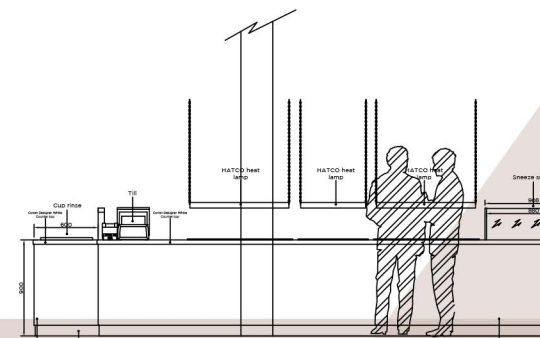
ELEVATION BB
