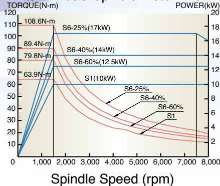
8,000rpm HEIDENHAIN QAN-200U Spindle Motor #40
