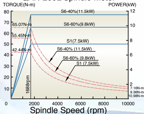
10,000rpm HEIDENHAIN QAN-200L Spindle Motor
