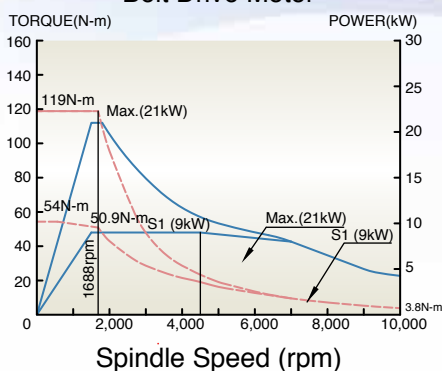
10,000rpm HEIDENHAIN QAN-200L Spindle Motor
