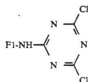
(DTAF)2,4-dichloro-1,3,5-triazin-2-ylamino-fluorescein
