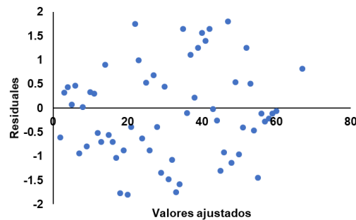
Figura 2. Estimación de Volumen en arboles individuales de Pinus hartwegii en el oriente del Valle de México, México. a) Curva ajustada con el modelo de regresión, y b) Distribución de residuales.
