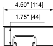
JAMB, 4 1/2" 6063-T6
