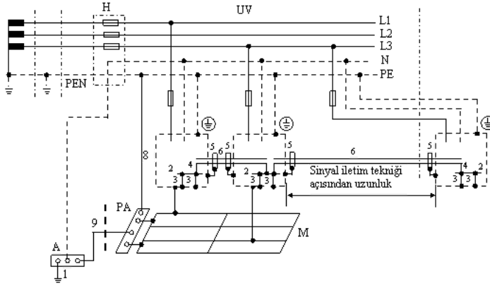
Şekil-25 Aynı alt dağıtım panosundan beslenen uzaktaki bir son cihaza sahip iletişim tesislerinin topraklamasına örnek (Not: Bu şekil mecburi olmayıp, yalnızca bir fikir vermek amacıyla taşınmaktadır.)
