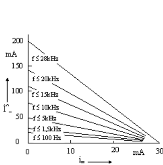
Şekil-Y.3 Boyutlandırma sınıfı 2'de izin verilen akım değerleri
