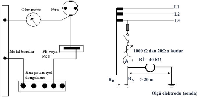
Şekil-8a Koruma iletkenlerinin bağlantısının ölçülmesi
