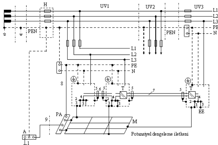
Şekil-26 Aynı şebeke beslemeli, ekranlı iletim hatlı ve ayrı topraklama veya potansiyel dengeleme tesisine sahip iletişim tesislerinin topraklamasına örnek (Not: Bu şekil mecburi olmayıp, yalnızca bir fikir vermek amacıyla taşınmaktadır.)
