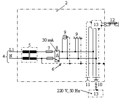
Şekil-30 Madde 28-d2'de belirtilen, bir fazlı alternatif akıma bağlı, ayırma transformatörlü, aşırı akım ve hata akımı koruma düzenleri ve potansiyel dengelmesi bulunan bir sinyal iletim tesisine örnek (Not: Bu şekil mecburi olmayıp, yalnızca bir fikir vermek amacıyla taşınmaktadır.)
