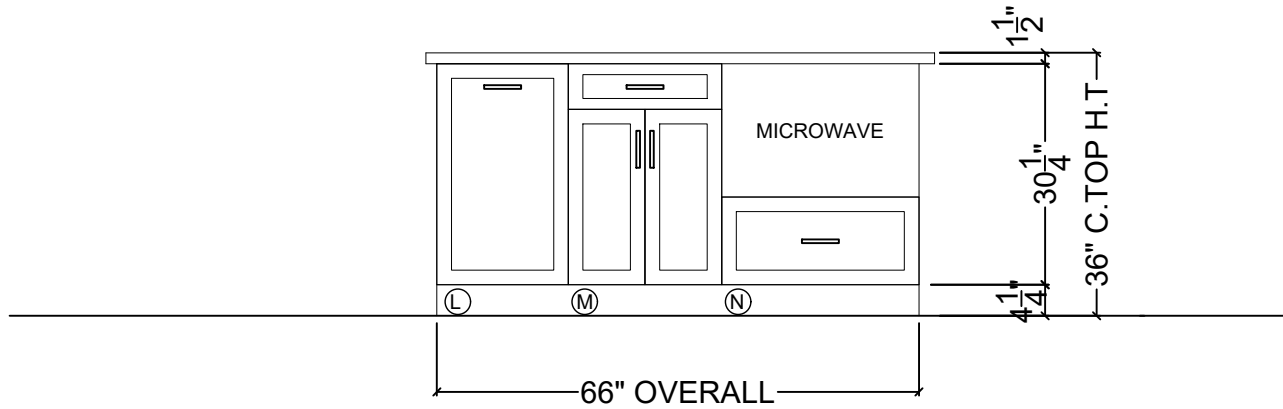
E3 KITCHEN ELEVATION
