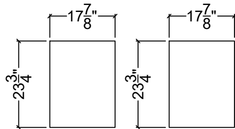
LEFT HINGE DOOR RIGHT HINGE DOOR
