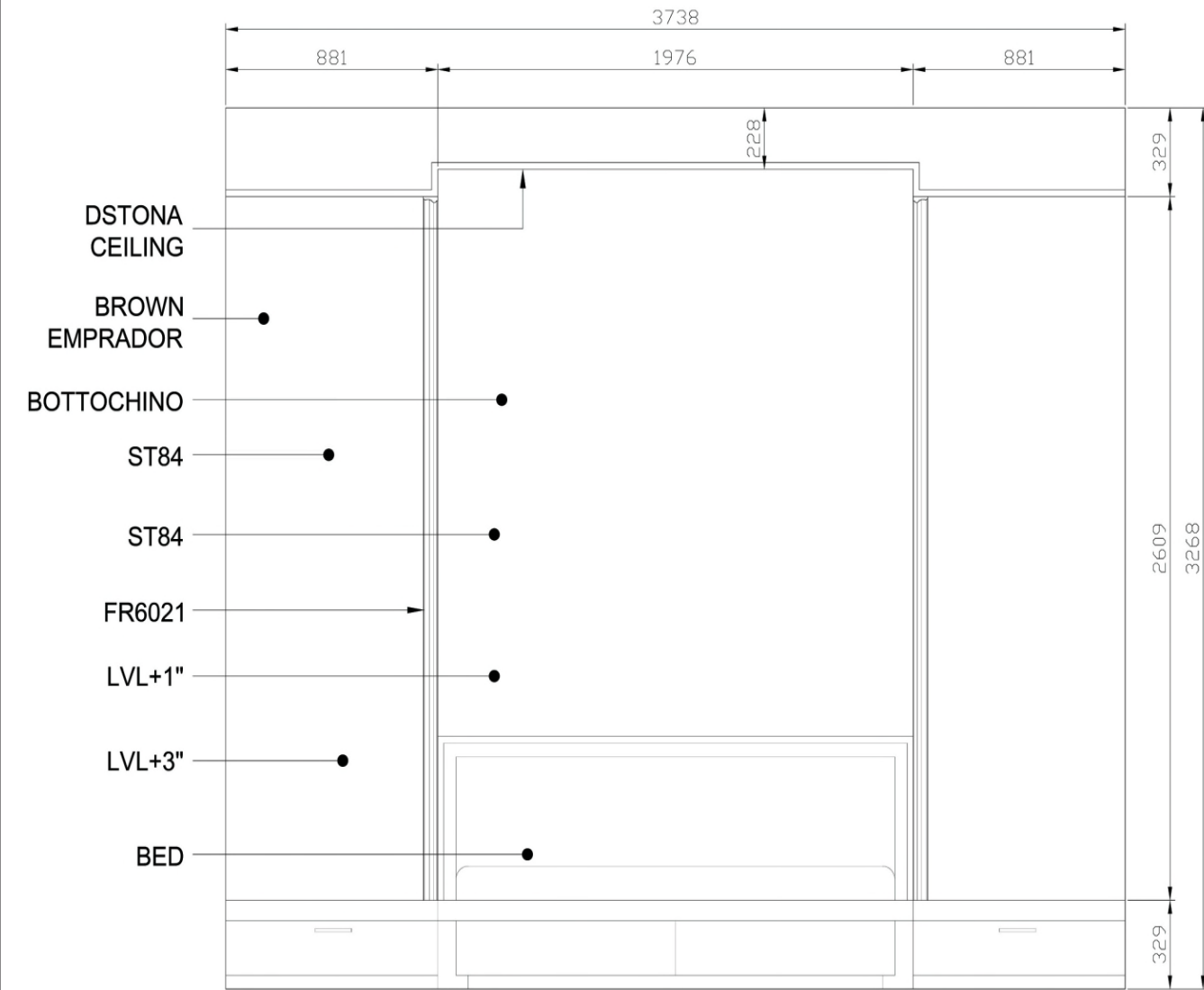
ELEVATION
