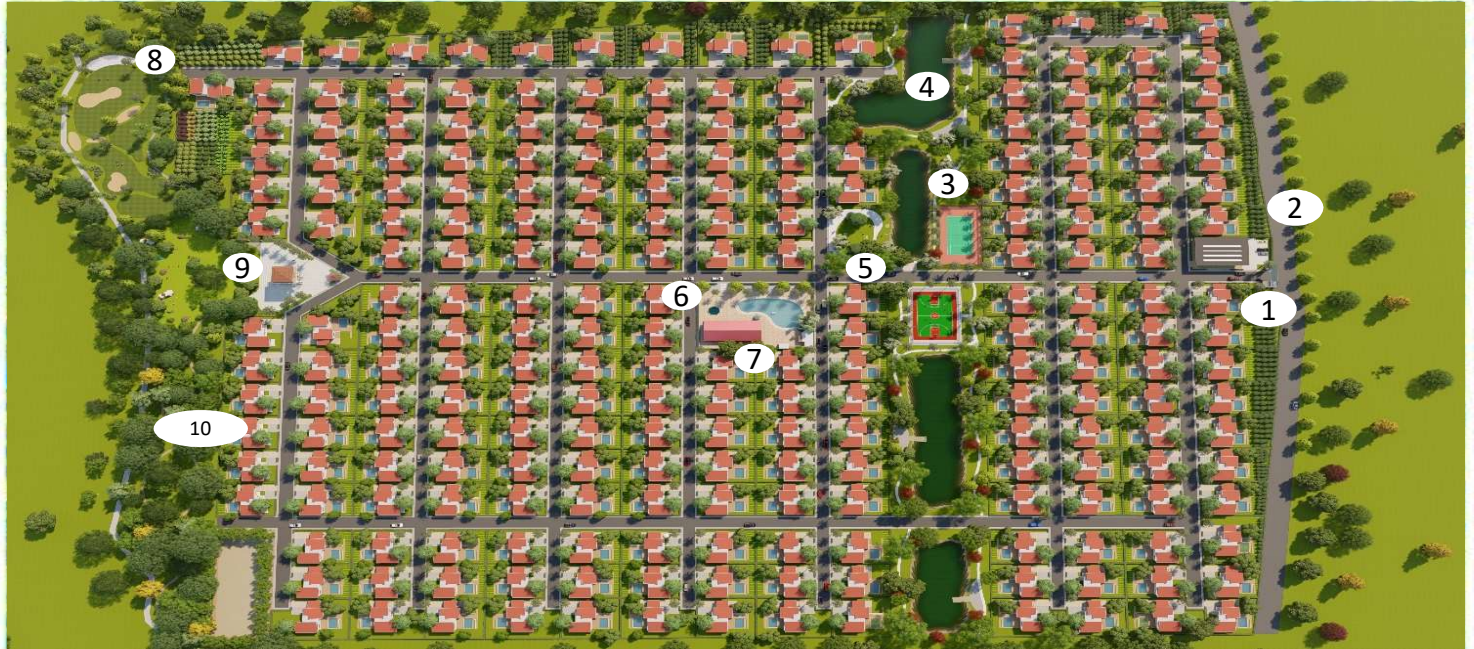
10. SENDEROS ECOLÓGICOS
