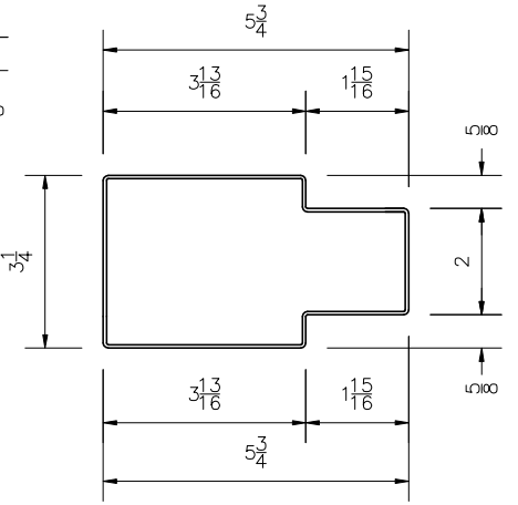
SR-MULLION
