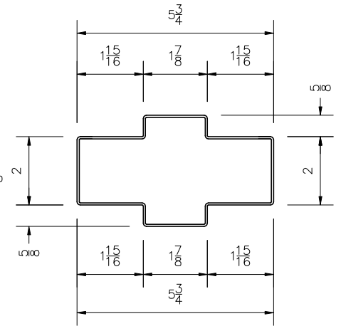
DR-MULLION
