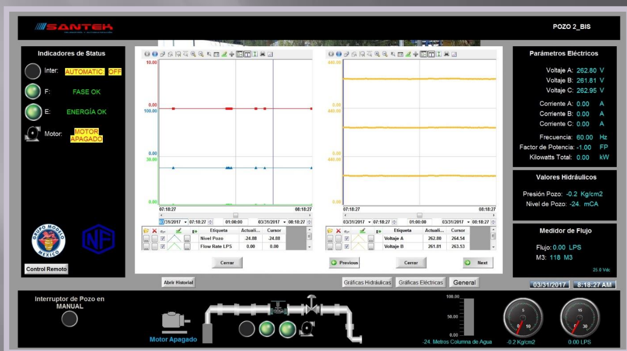
Pantalla graficas de Telemetría SCADAGRAPH 3000 2 WAVE
