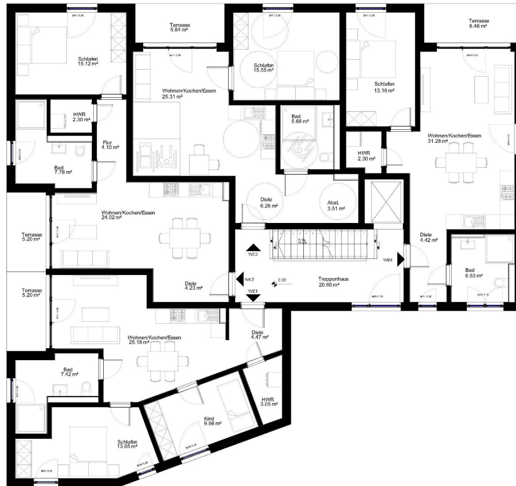
GRUNDRISS ERDGESCHOSS
