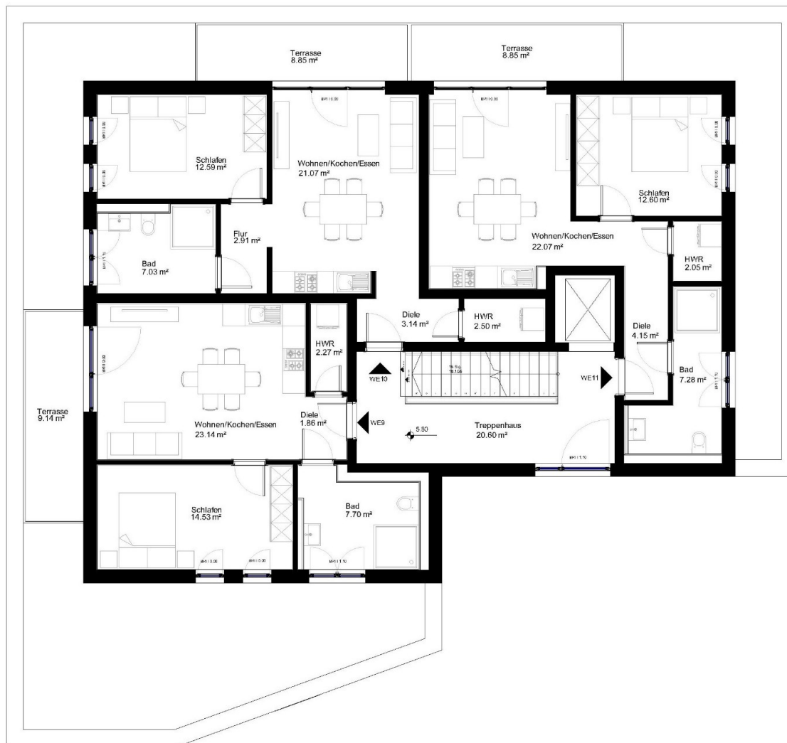
GRUNDRISS STAFFELGESCHOSS
