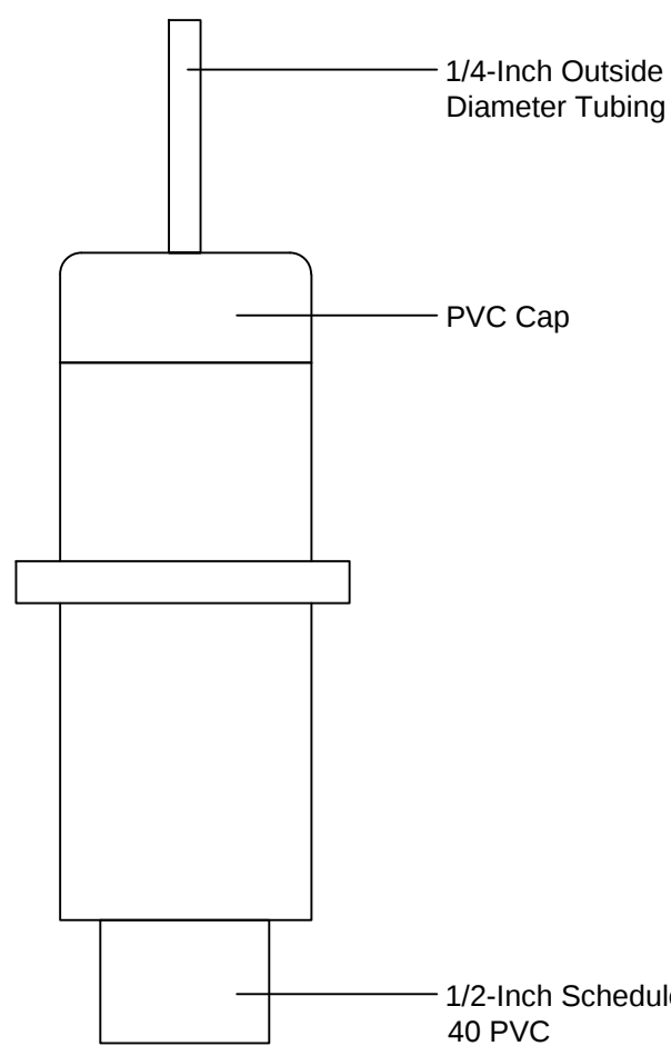
AMB VENT RISER PRESSURE TEST PORT No Scale
