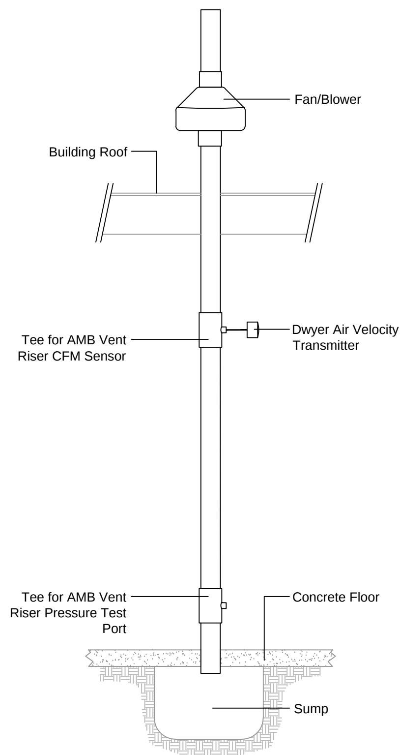
AMB VENT RISER MONITORING EQUIPMENT No Scale
