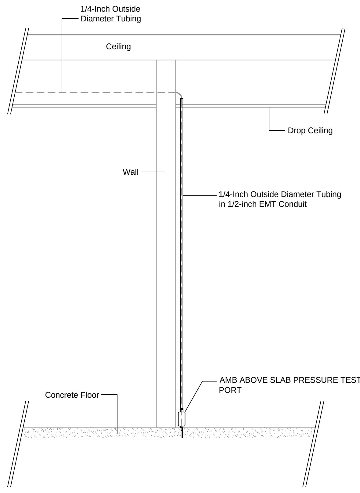
AMB ABOVE SLAB TEST PORT ROUTING No Scale
