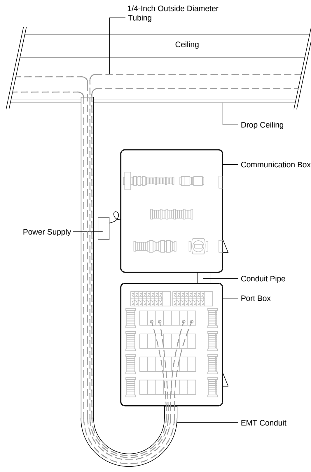
AMB VAPOR MONITORING TELEMETRY SYSTEM WALL BOXES No Scale
