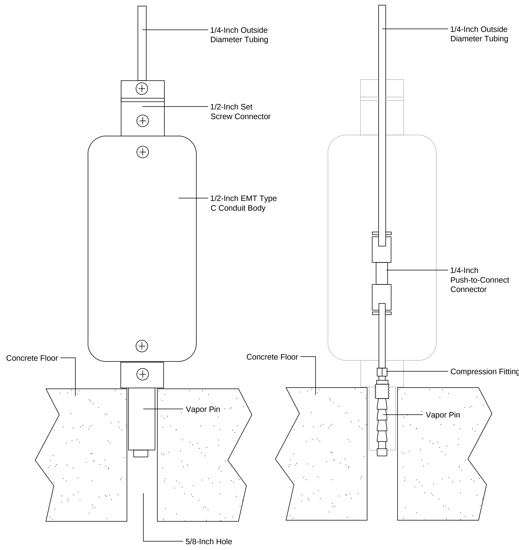
AMB ABOVE SLAB PRESSURE TEST PORT No Scale
