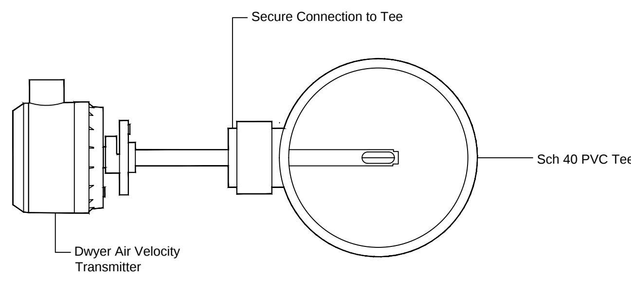
AMB VENT RISER CFM SENSOR No Scale
