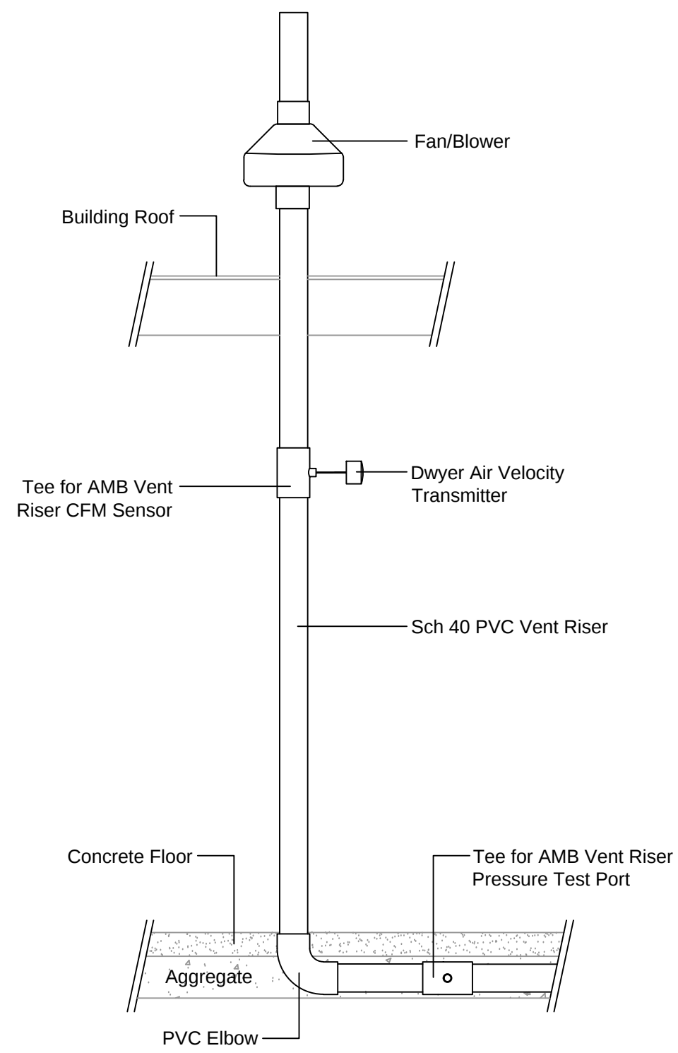
VENT RISER WITH AMB VAPOR MONITORING EQUIPMENT No Scale
