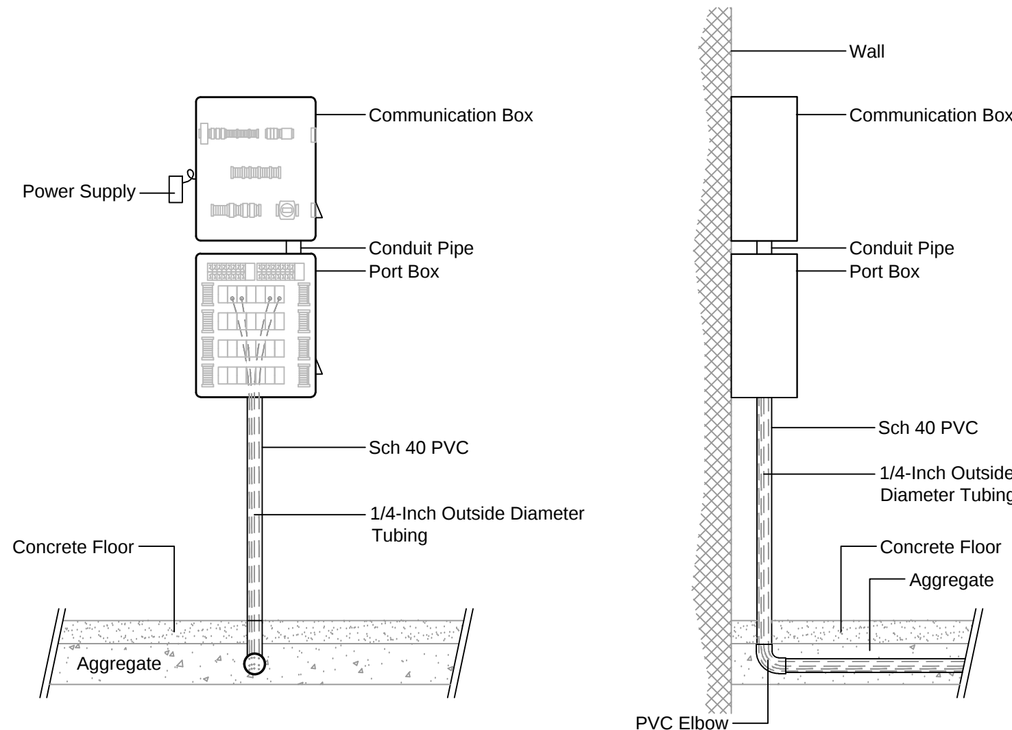
AMB VAPOR MONITORING TELEMETRY SYSTEM WALL BOXES No Scale
