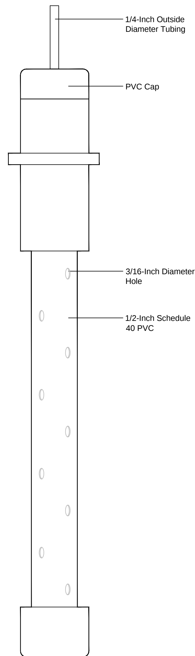
AMB BELOW SLAB PRESSURE TEST PORT No Scale
