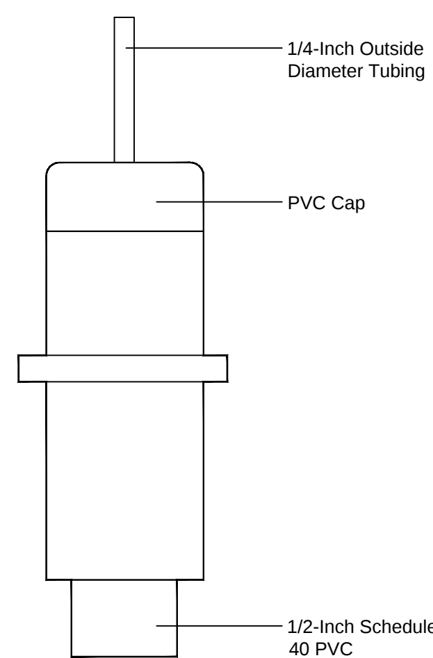
AMB VENT RISER PRESSURE TEST PORT No Scale
