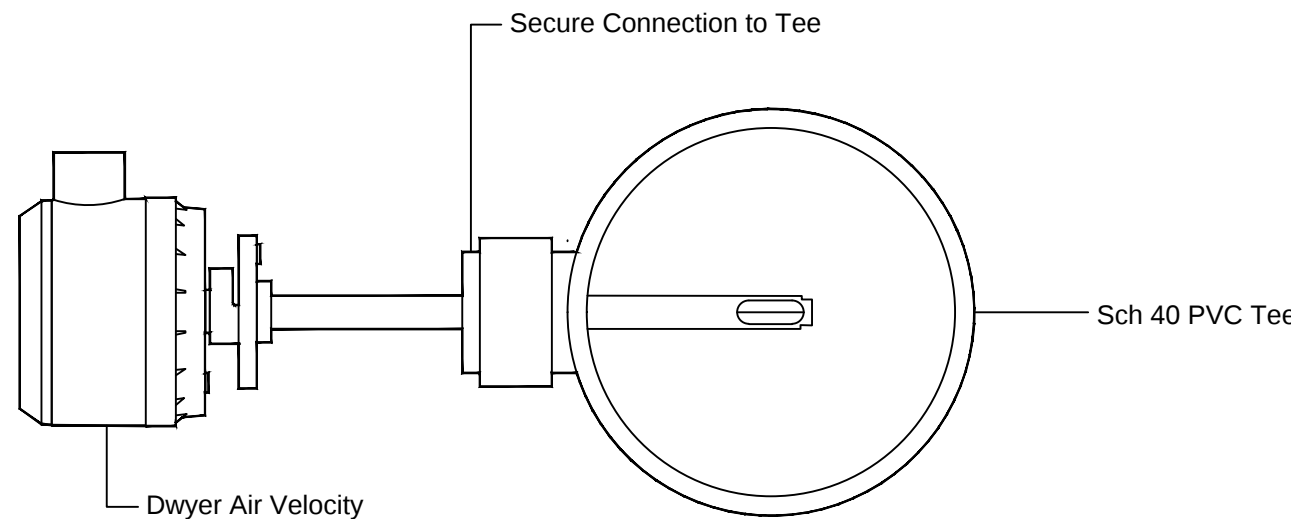
AMB VENT RISER CFM SENSOR No Scale
